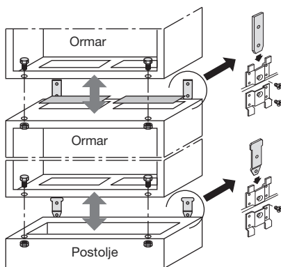
Vertikalno spajanje ormara IP 44 / IP 54
